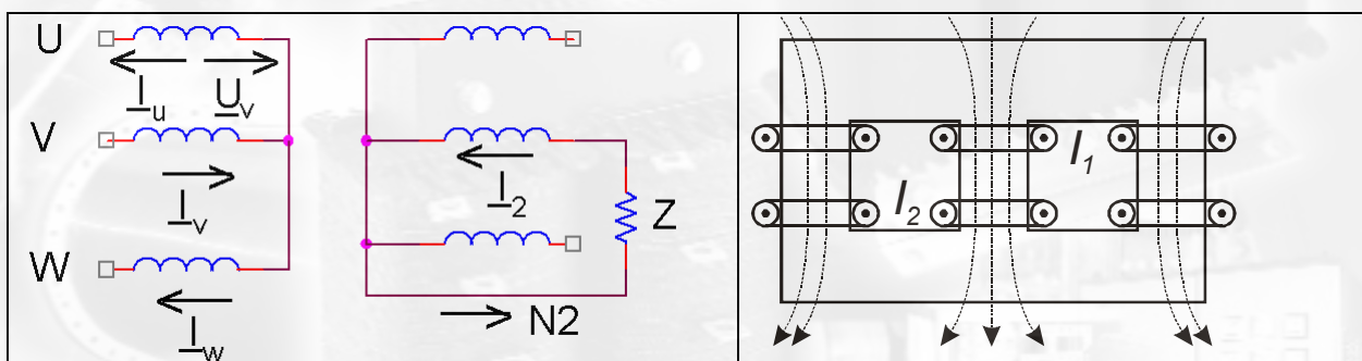
Bild 3.2.4: Einsträngige Belastung bei Schaltgruppe Yyn
